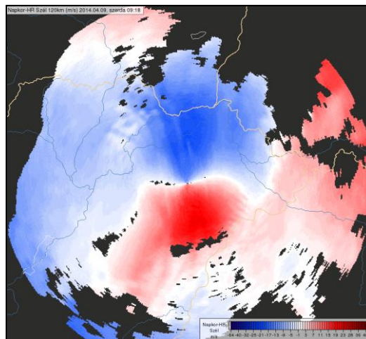
4. ábra. Doppler radiális szélmérés 1,1^\circ -os magassági szögön. A kék szín a radarhoz közeledő, a piros a radartól távolodó mozgásra utal. Jelen esetben északias irányú a szél a radar szűk környezetében, de ahogy egyre magasabban mérünk (távolodva a radartól) szélfordulás figyelhető meg.
