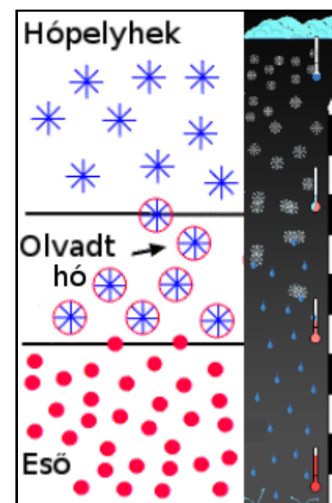
14. ábra. Az olvadási rétegben a hópehelyek elkezdnek megolvadni, így vízréteg burkolja őket, azonban méretük ekkor még nagyobb, mint a teljes megolvadás után az esőcseppeké.
